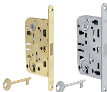
Magnetica foro chiave "Magnetica!" key hole
